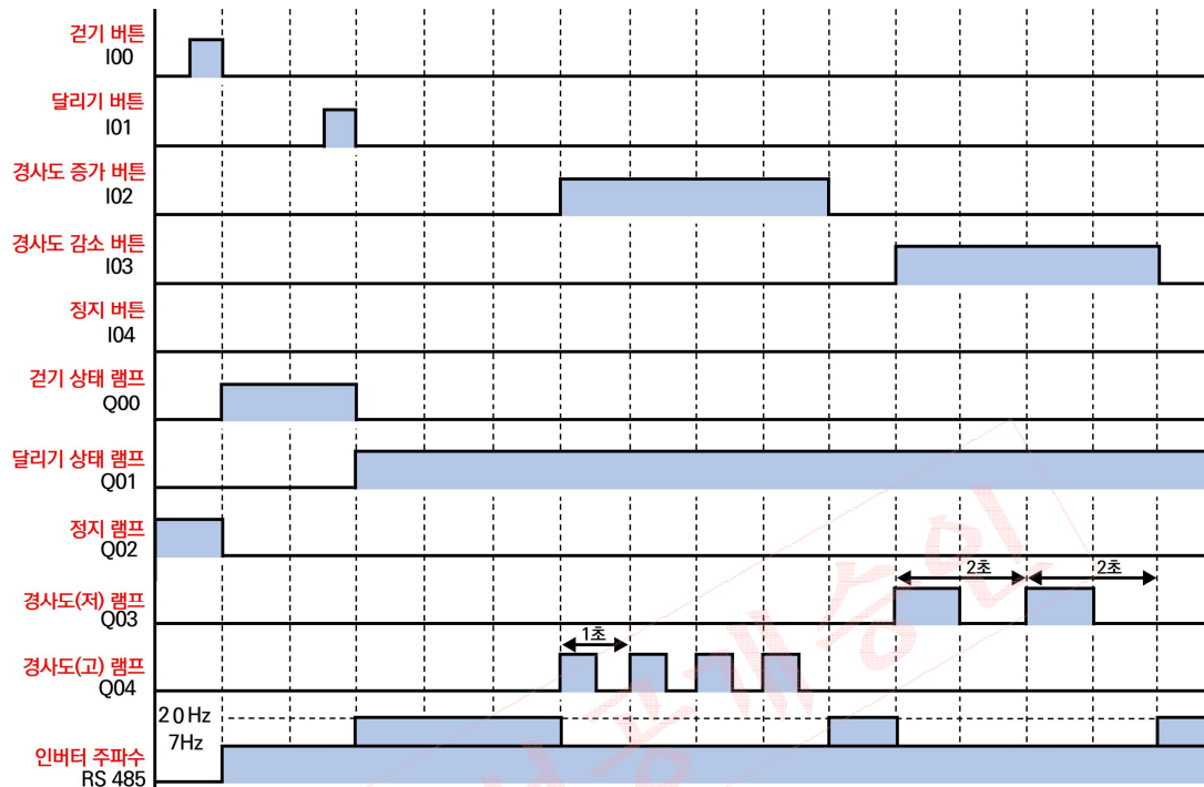
[견기, 달리기 / 경사도 증가, 감소 동작_견기, 달리기]
